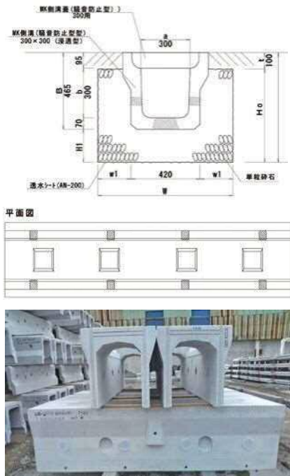
浸透側溝 施工例
