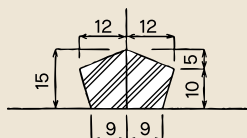
目地部詳細図(モルタル目地)
