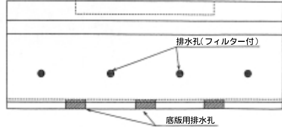
側面図
